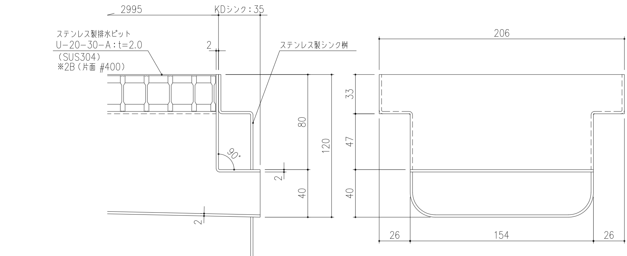
接続部詳細図 S=1/2
