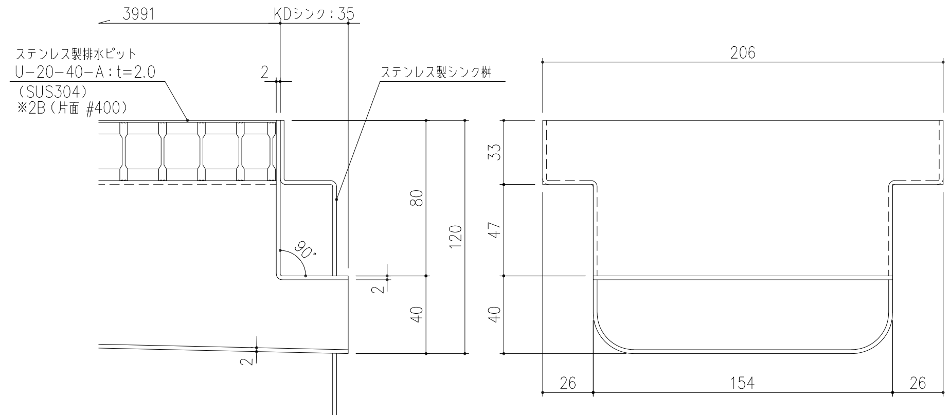
接続部詳細図 S=1/2
