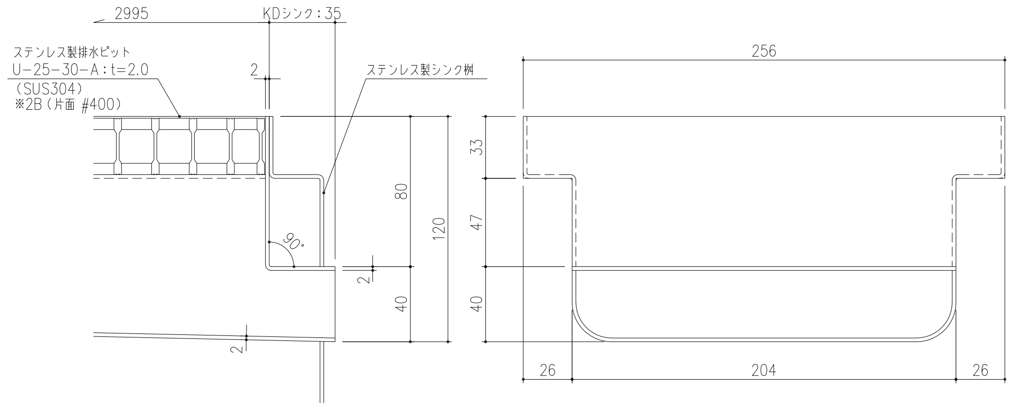
接続部詳細図 S=1/2
