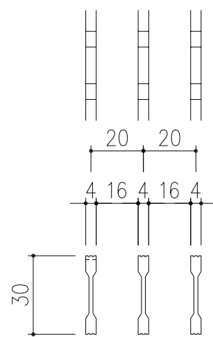
メインバーピッチ詳細図 S=1/2
