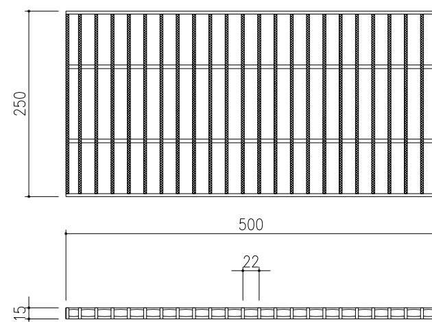
FR22-1525H 詳細図 S=/5
