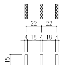
メンバーピッチ詳細図 S=1/2
