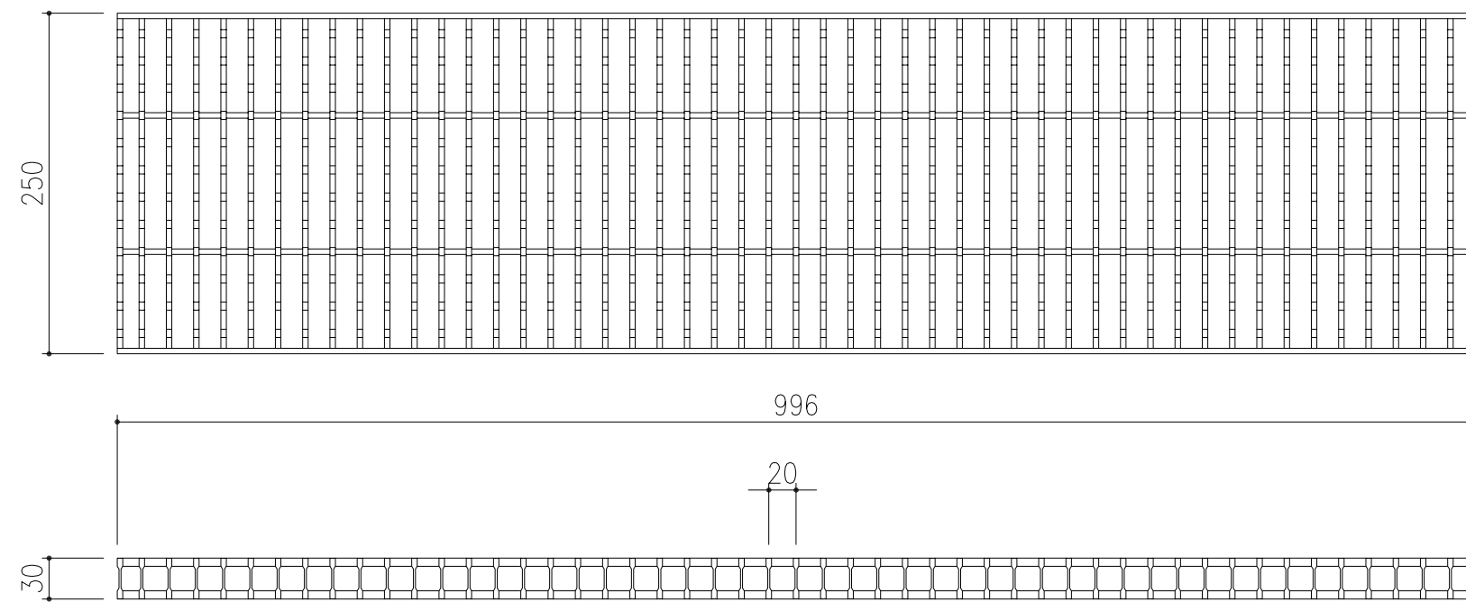
AG20-3025-2 詳細図 S= /5
