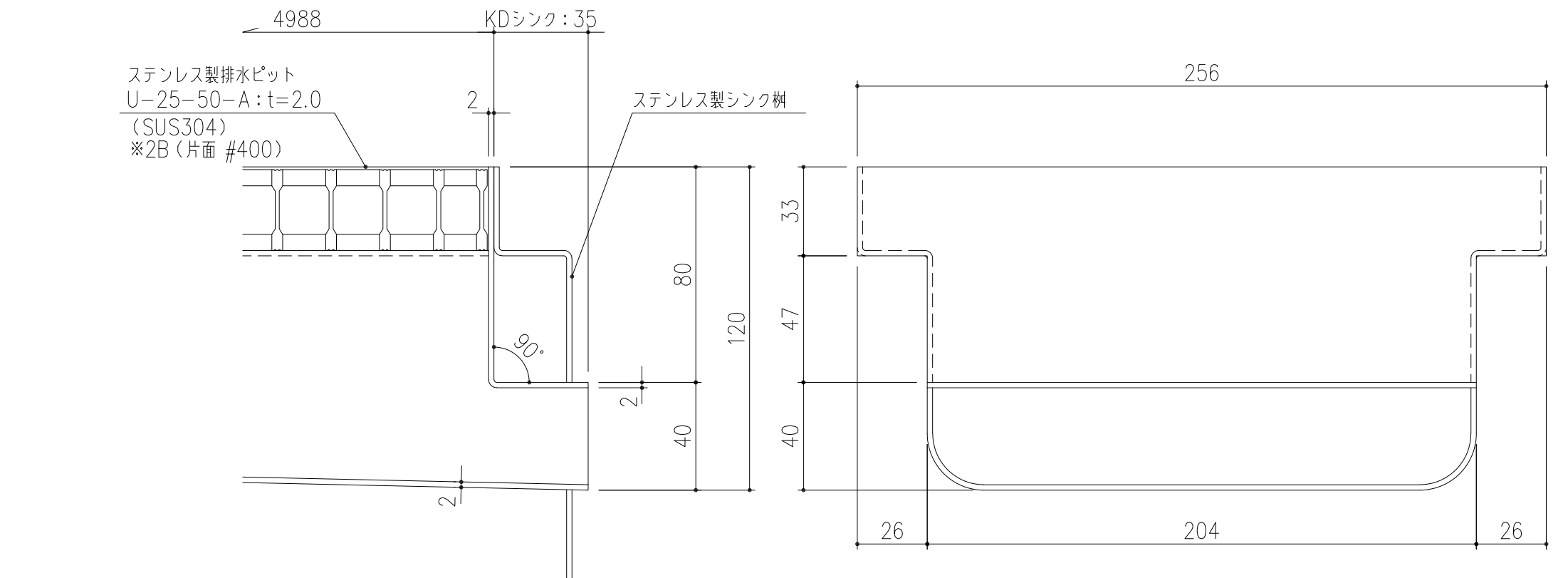
接続部詳細図 S=1/2
