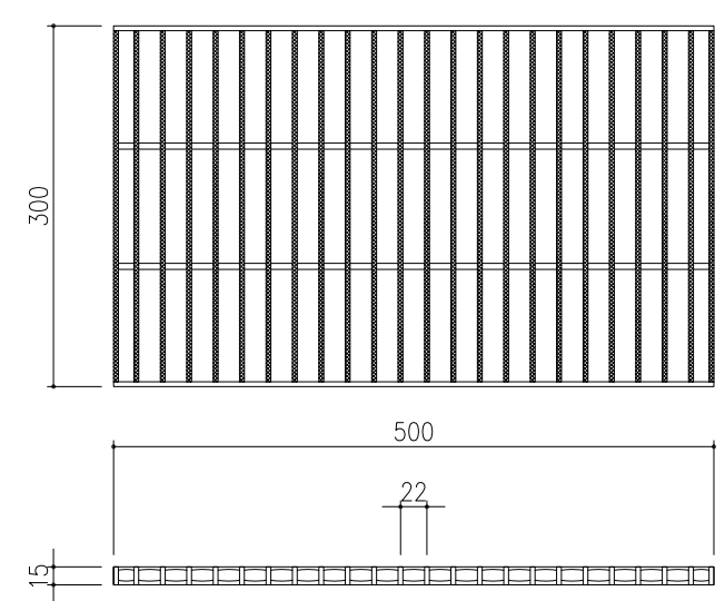
FR22-1530H 詳細図 S=1/5
