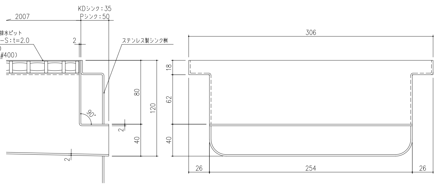
接続部詳細図 S=1/2
