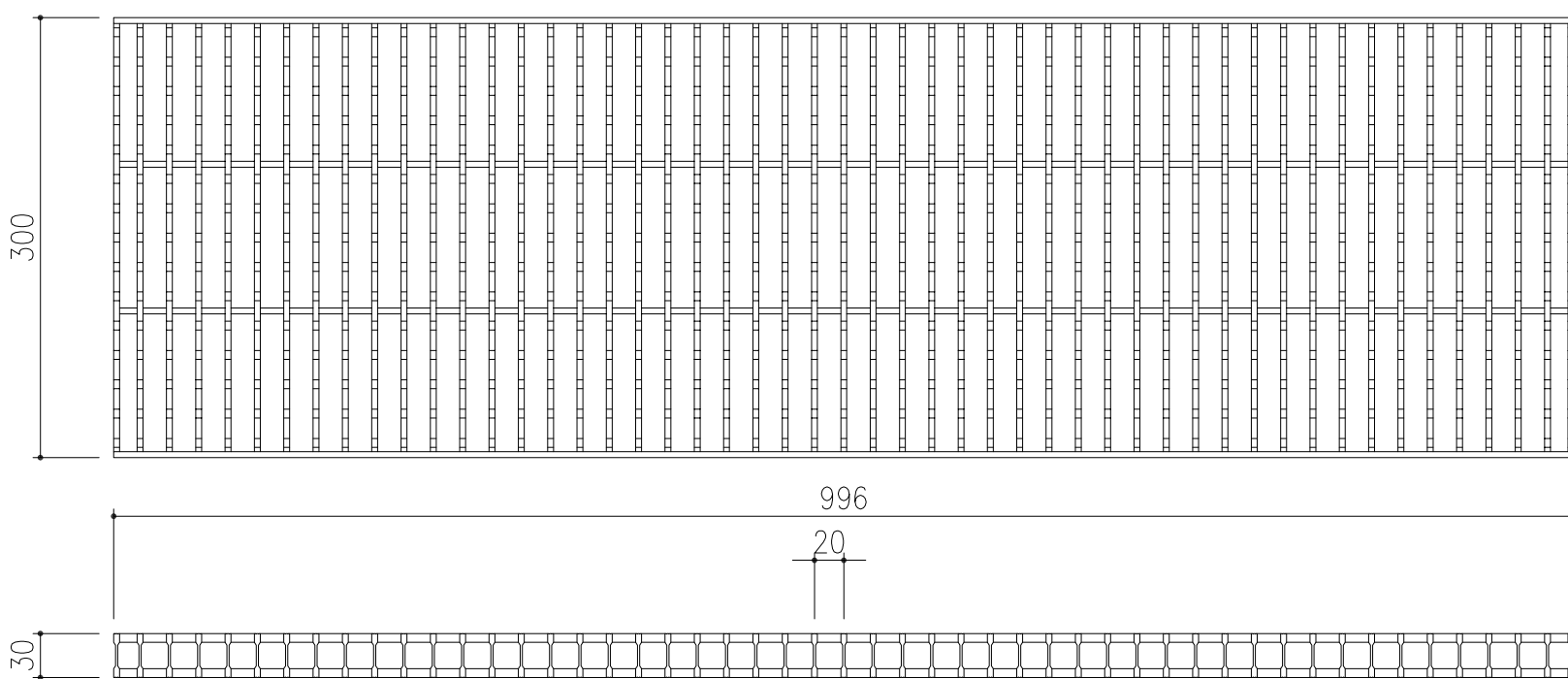
AG20-3030-2 詳細図 S=/5
