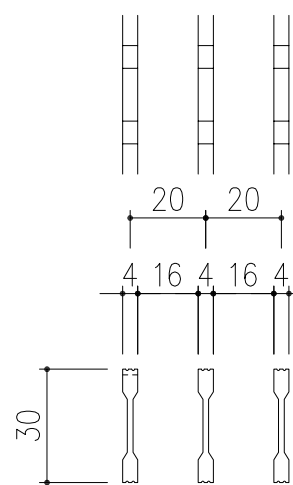
メンバーピッチ詳細図 S=1/2
