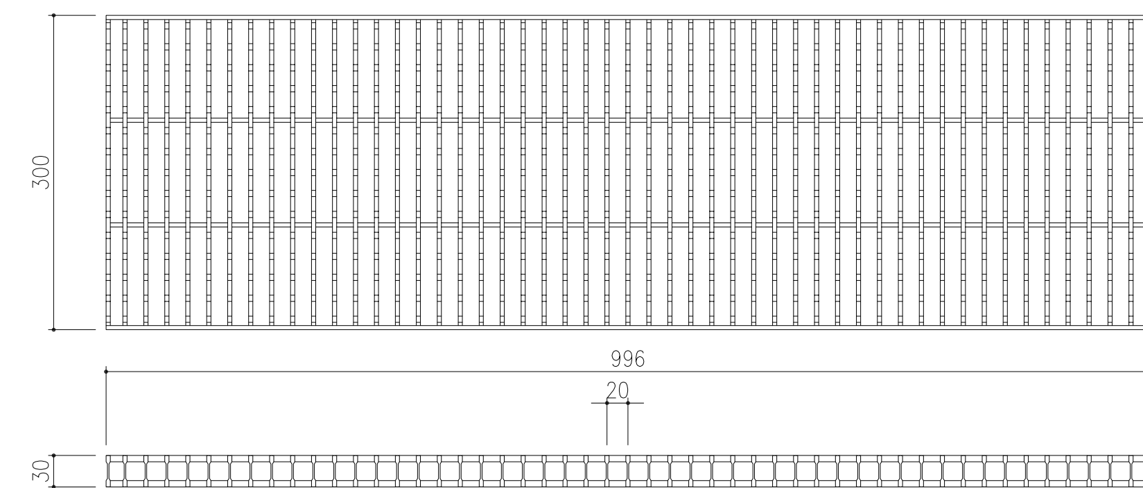
AG20-3030-2 詳細図 S= /5
