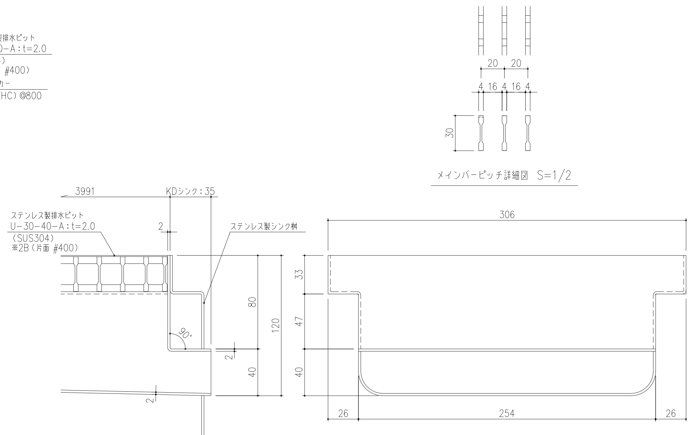
接続部詳細図 S=1/2
