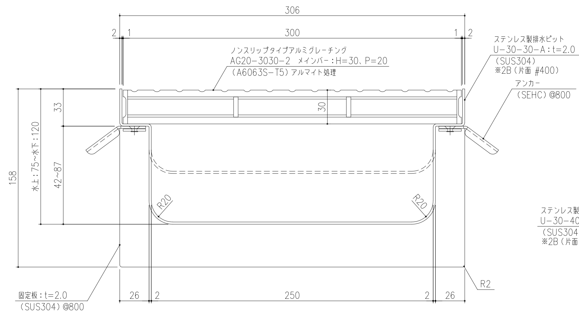
断面詳細図 S=1/2
