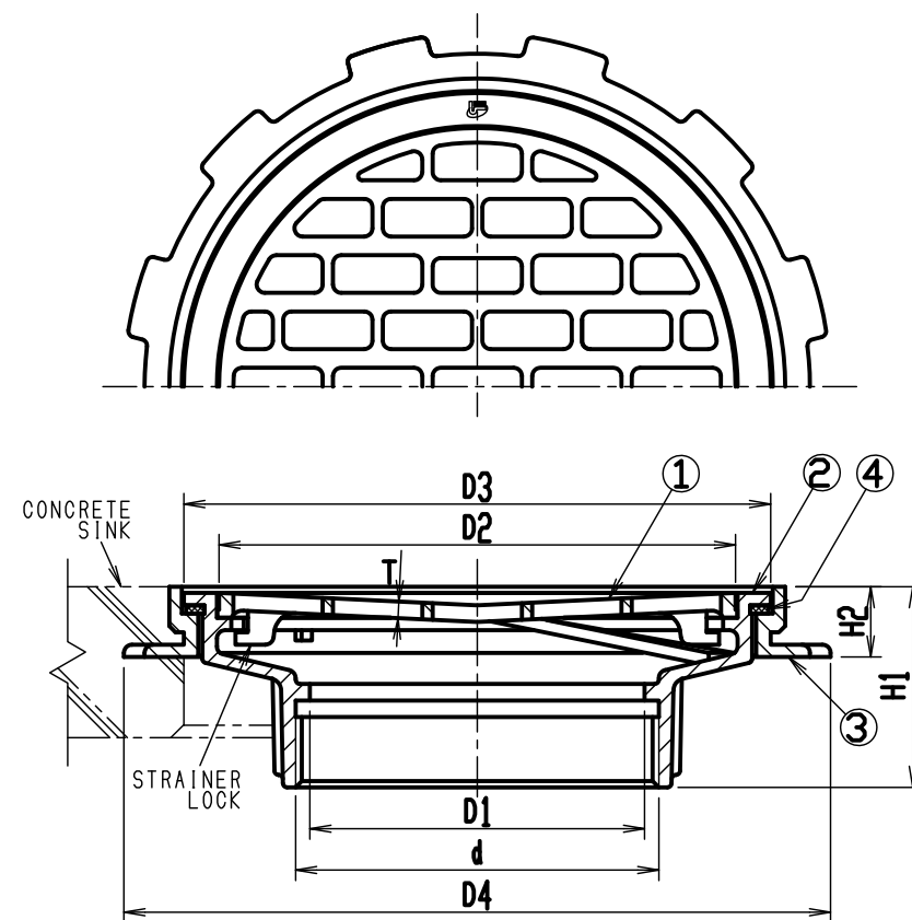
構成部品表
