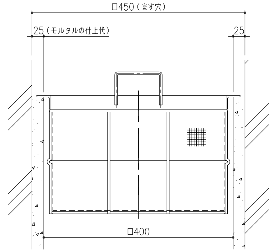
施工例
