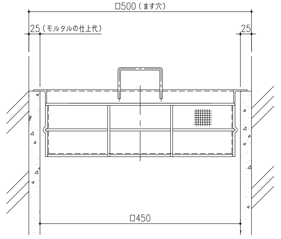
施工例
