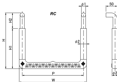
●寸法表 芯材:SWCH12R(芯材:SUS304)
