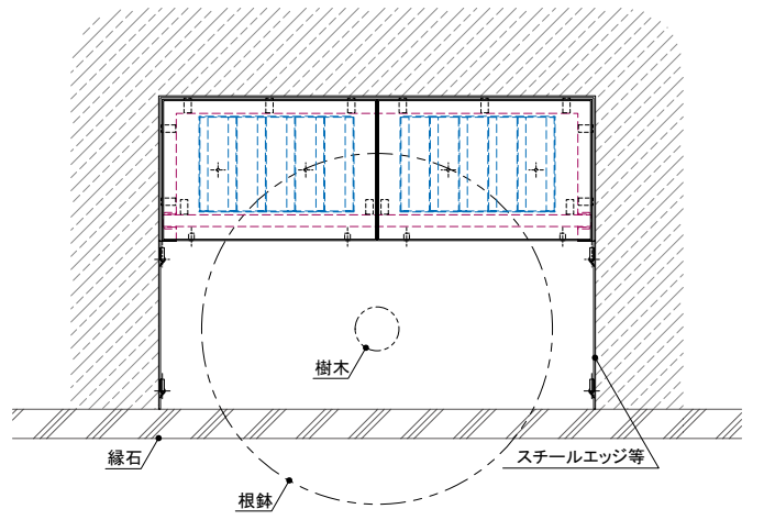
TPFF 使用例 (縁石)
