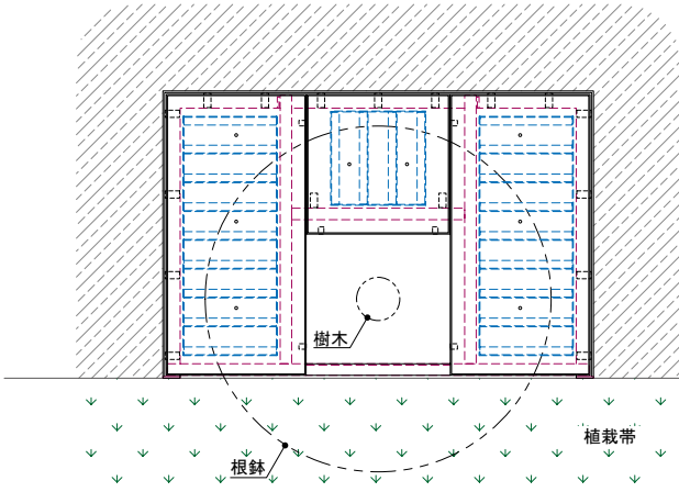
TPFF 使用例 (植栽帯)
