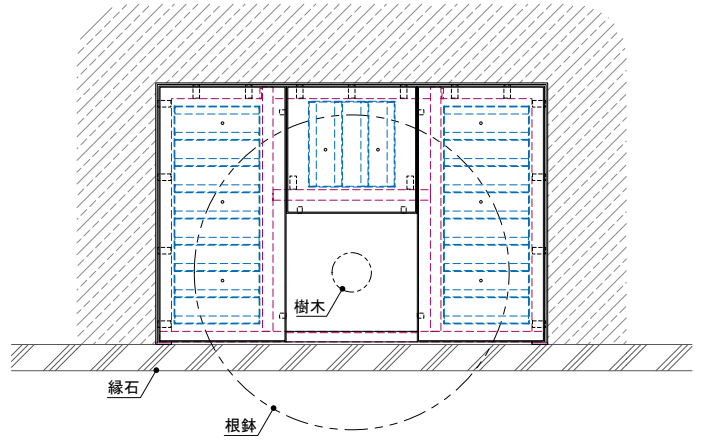
TPFF 使用例 (縁石)
