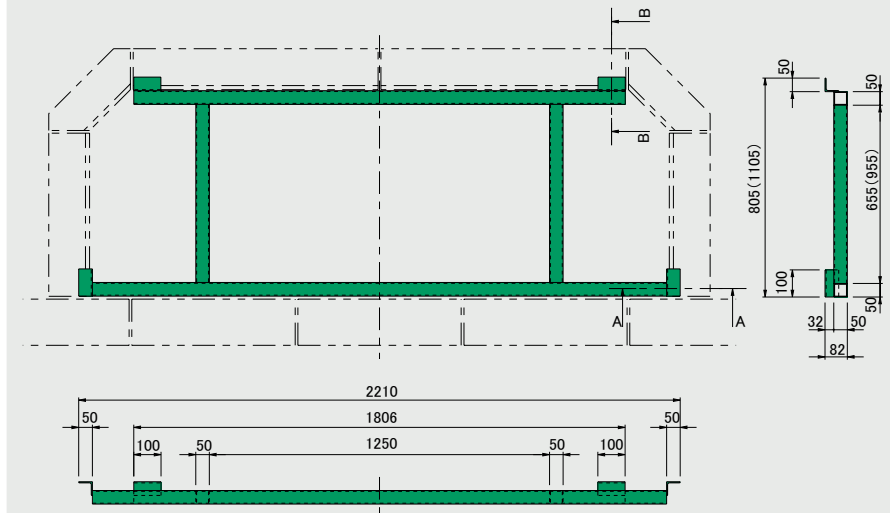
断面A-A
