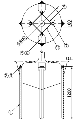
DJP-4M ●質量: 81kg
