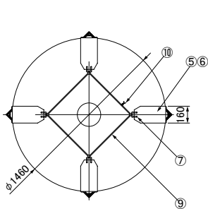
DJP-3 ●質量: 39kg
