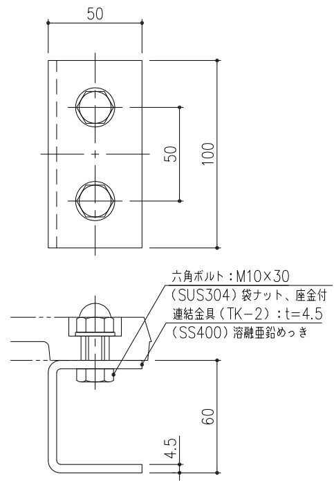
連結金具詳細図 S=1/2
