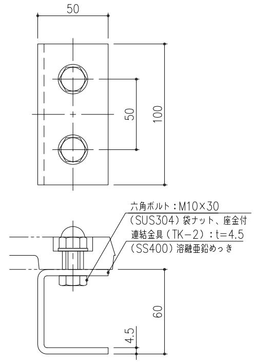
連結金具詳細図 S=1/2
