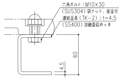
連結金具詳細図 S=1/2
