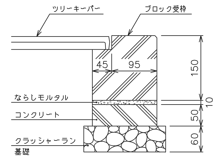
施工例 S=1/5
