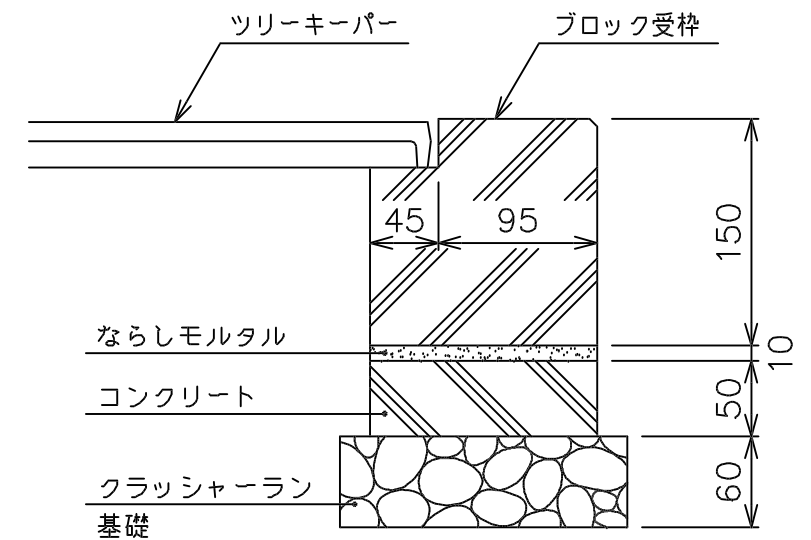
施工例 S=1/5
