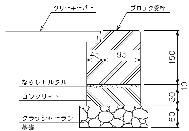
施工例 S=1/5
