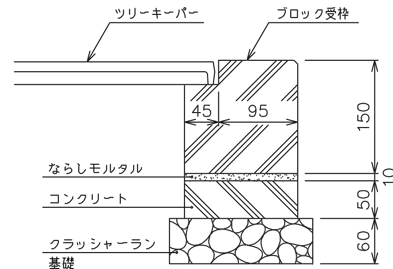
施工例 S=1/5
