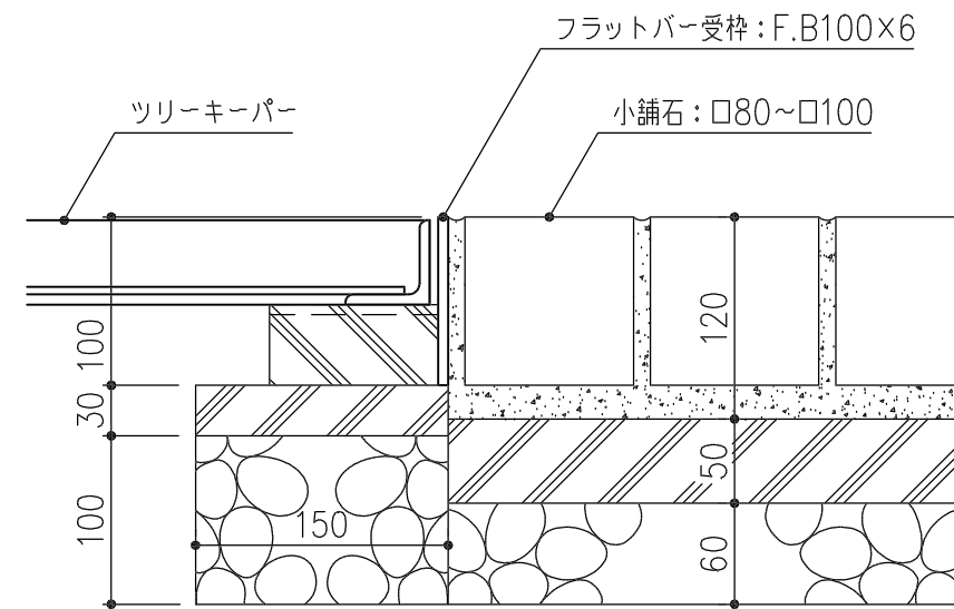
施工例 S=1/5
