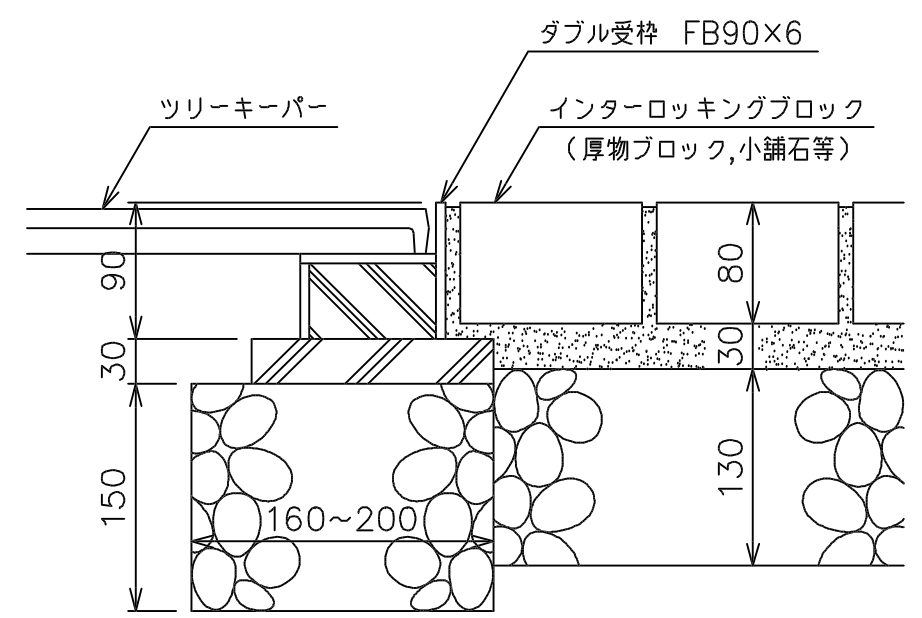
施工例 S=1/5
