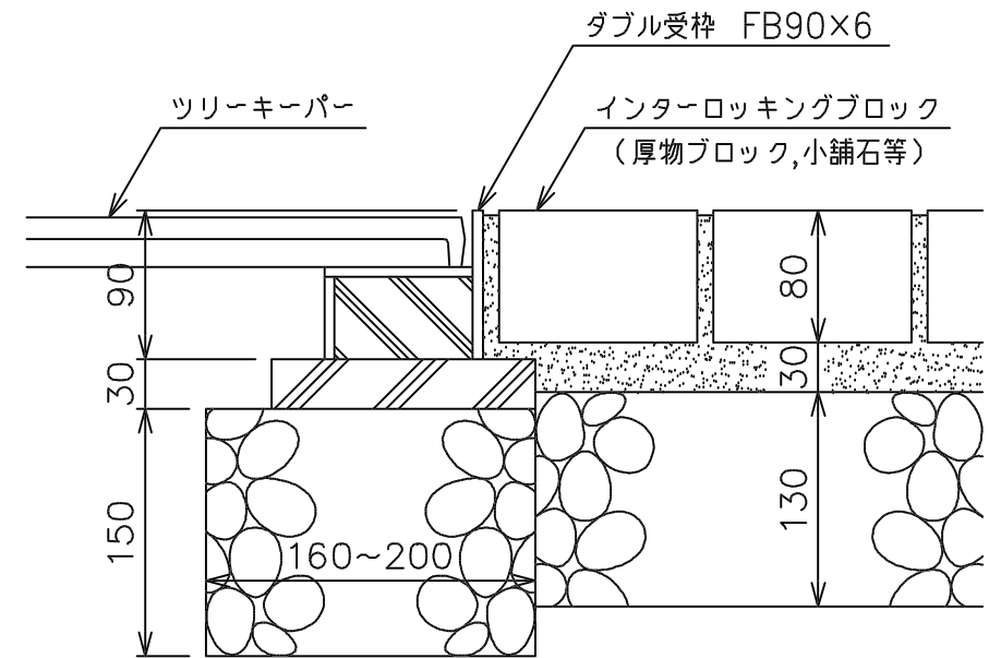
施工例 S=1/5
