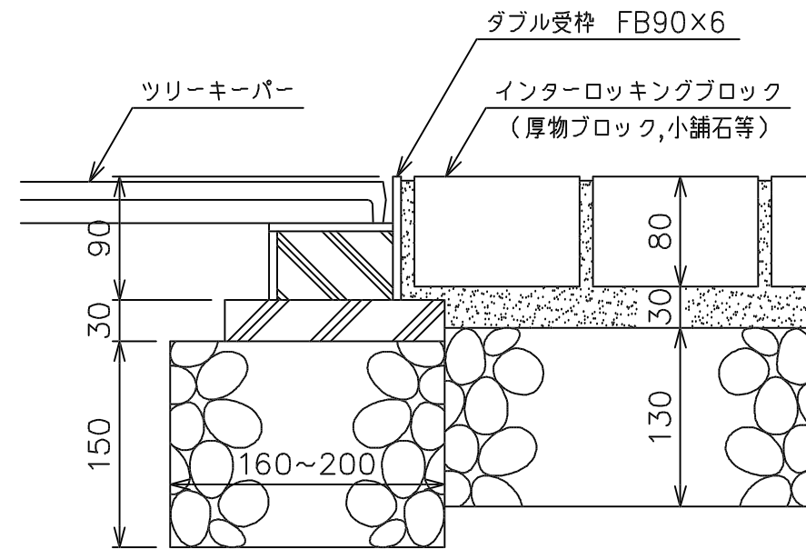
施工例 S=1/5
