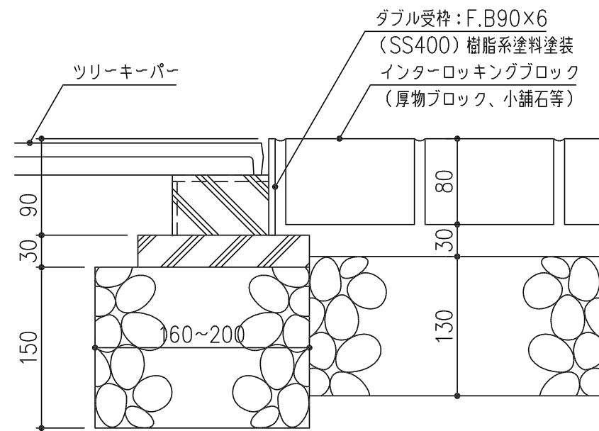
施工例 S=1/5
