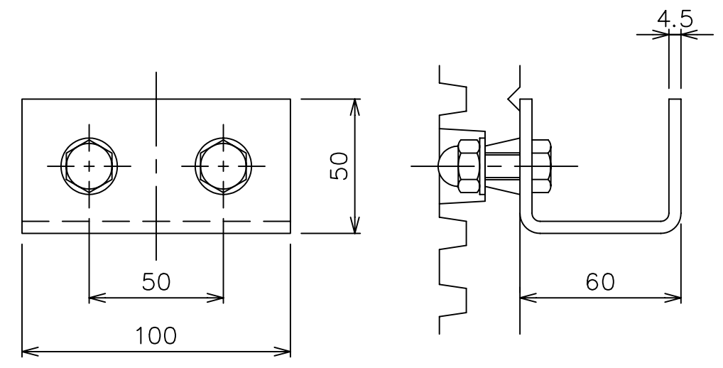
連結金具詳細図 S=1/2
