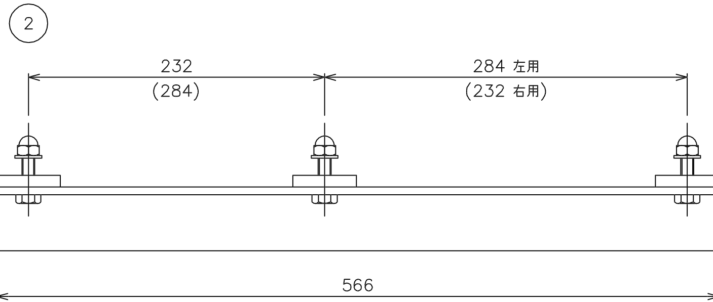
連結金具詳細図 S=1/3
