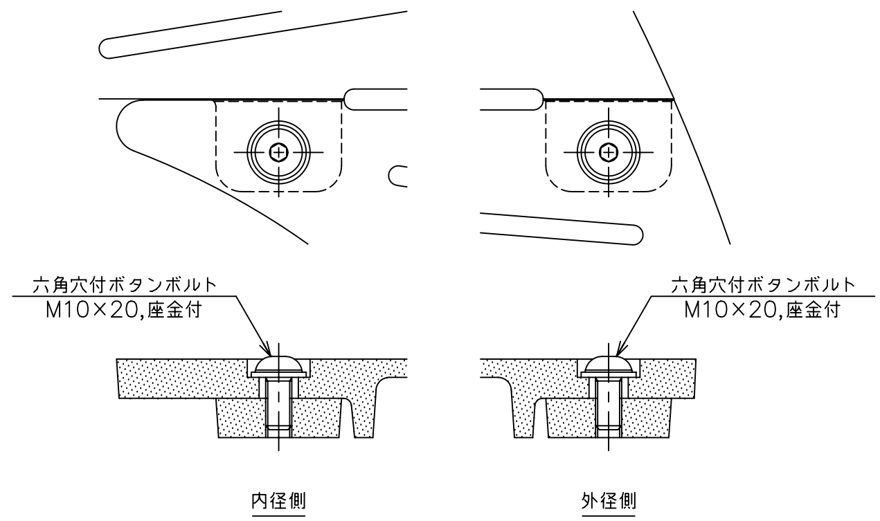
連結部詳細図 S=1/2
