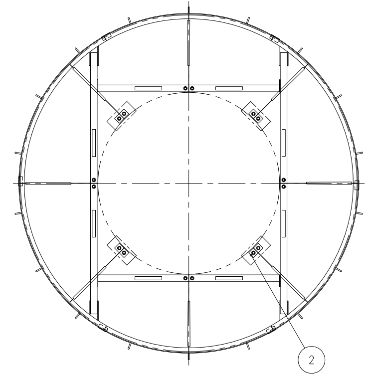
アングル補強受枠組合せ S=1/20
