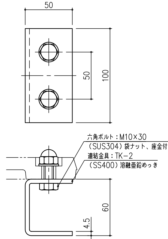
連結金具詳細図 S=1/2
