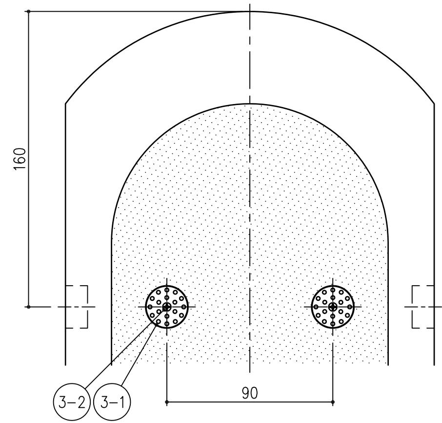
レфлекター詳細図 S=1/2
