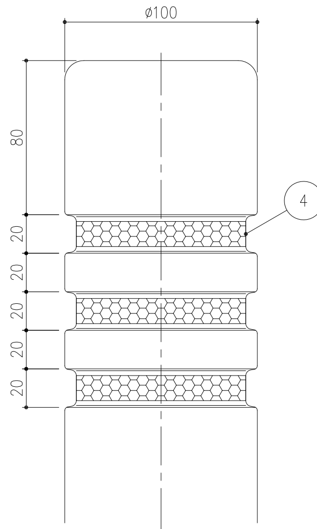
反射テープ詳細図 S=1/2
