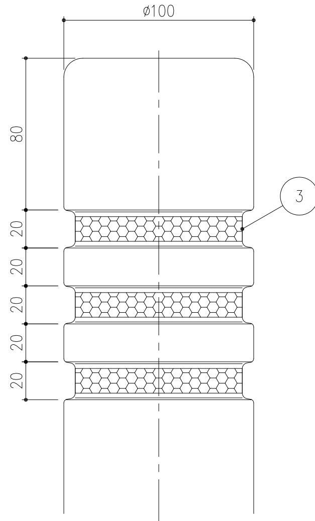
反射テープ詳細図 S=1/2
