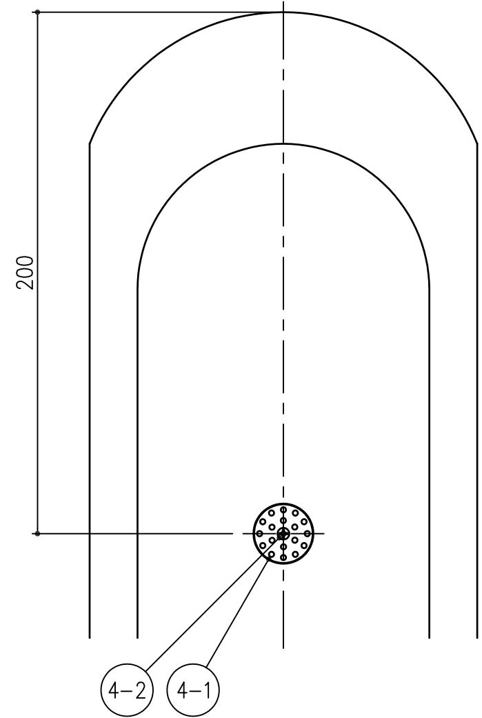
レфлекター詳細図 S=1/2
