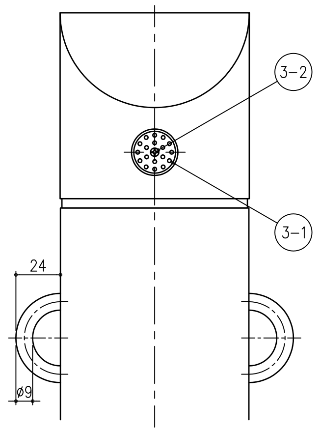
レフレクター詳細図 S=1/2
