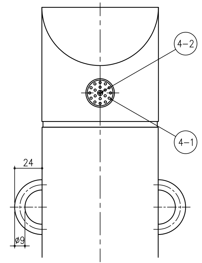
レфлекター詳細図 S=1/2
