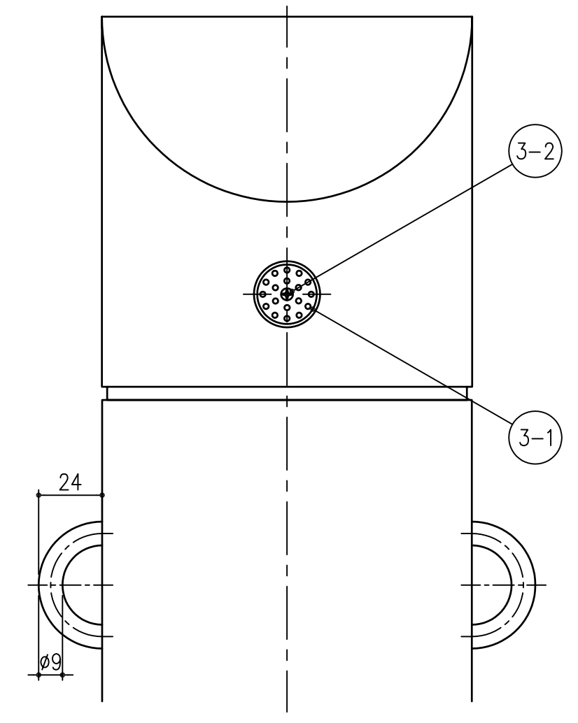
レフレクター詳細図 S=1/2
