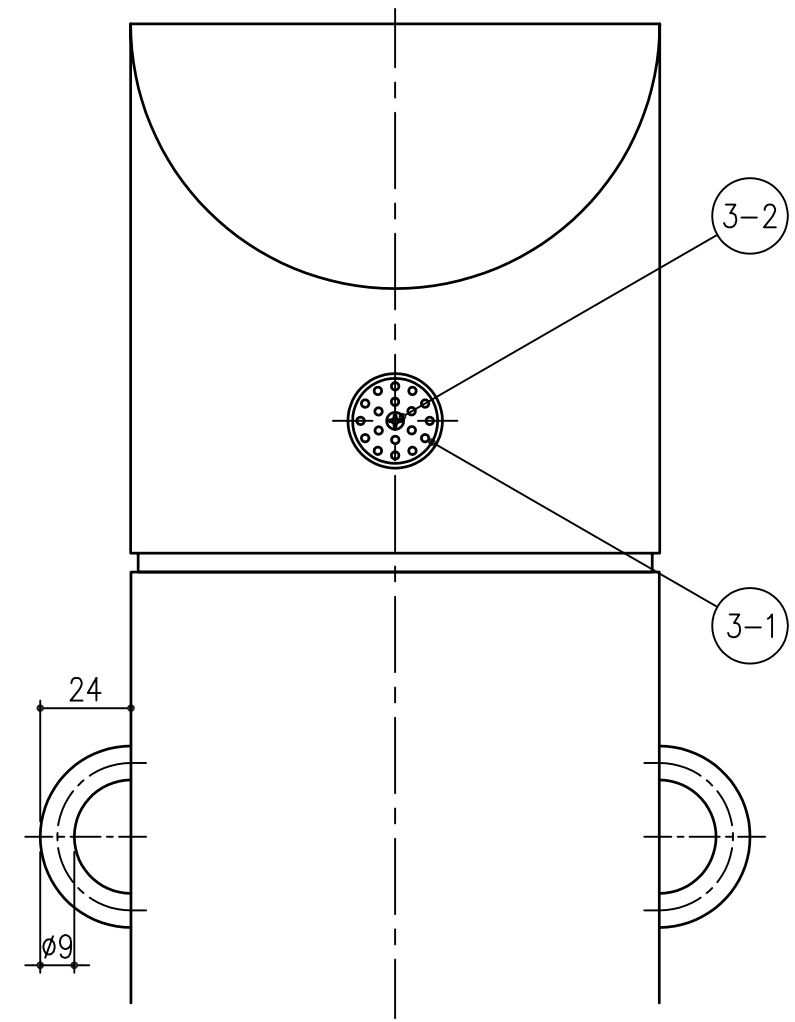
レフレクター詳細図 S=1/2
