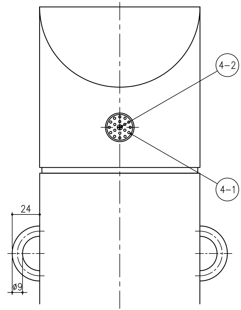
レфлекター詳細図 S=1/2
