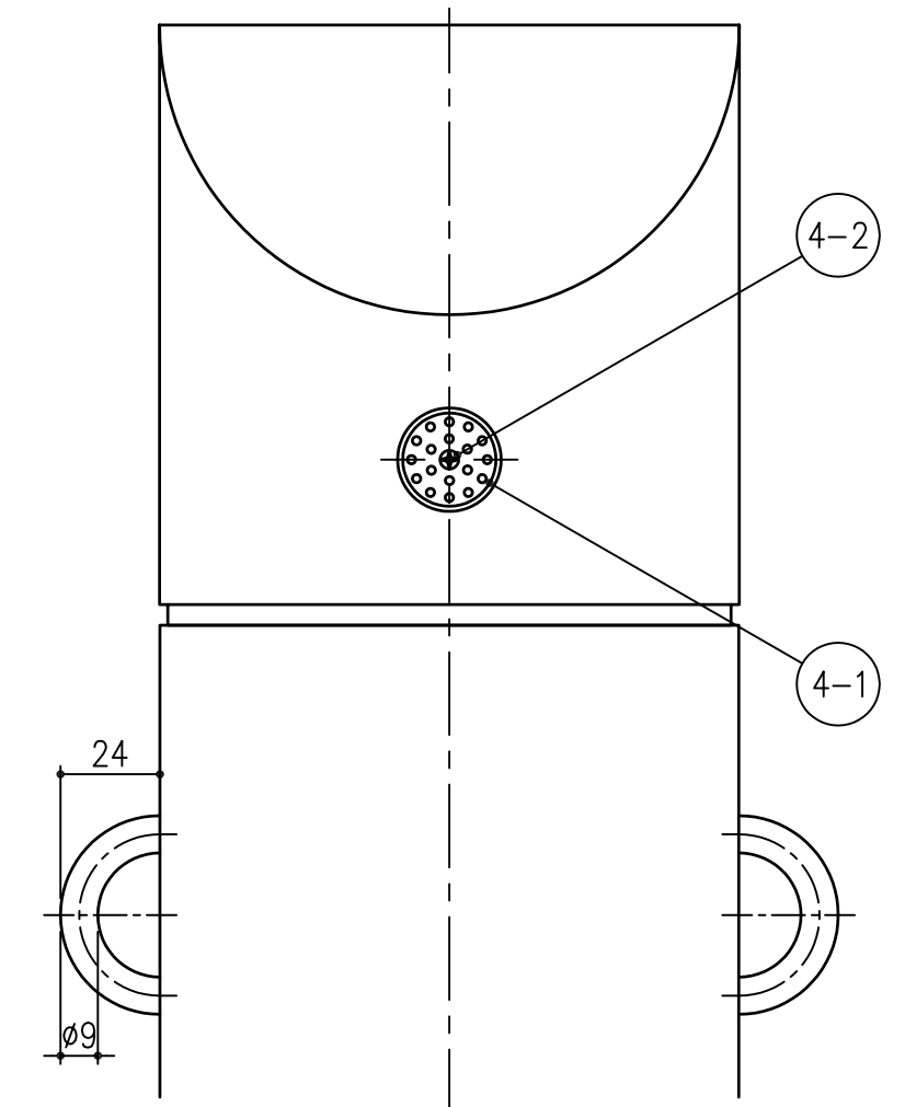
レфлекター詳細図 S=1/2
