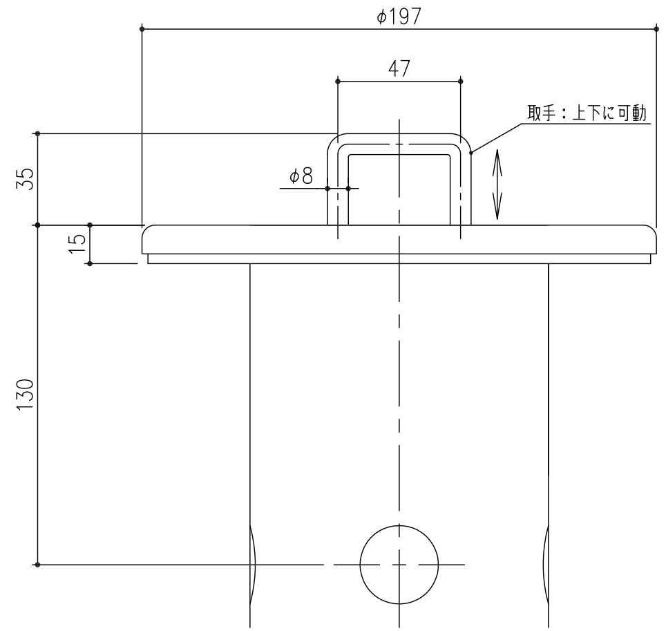
頭部詳細図 S=1/2
