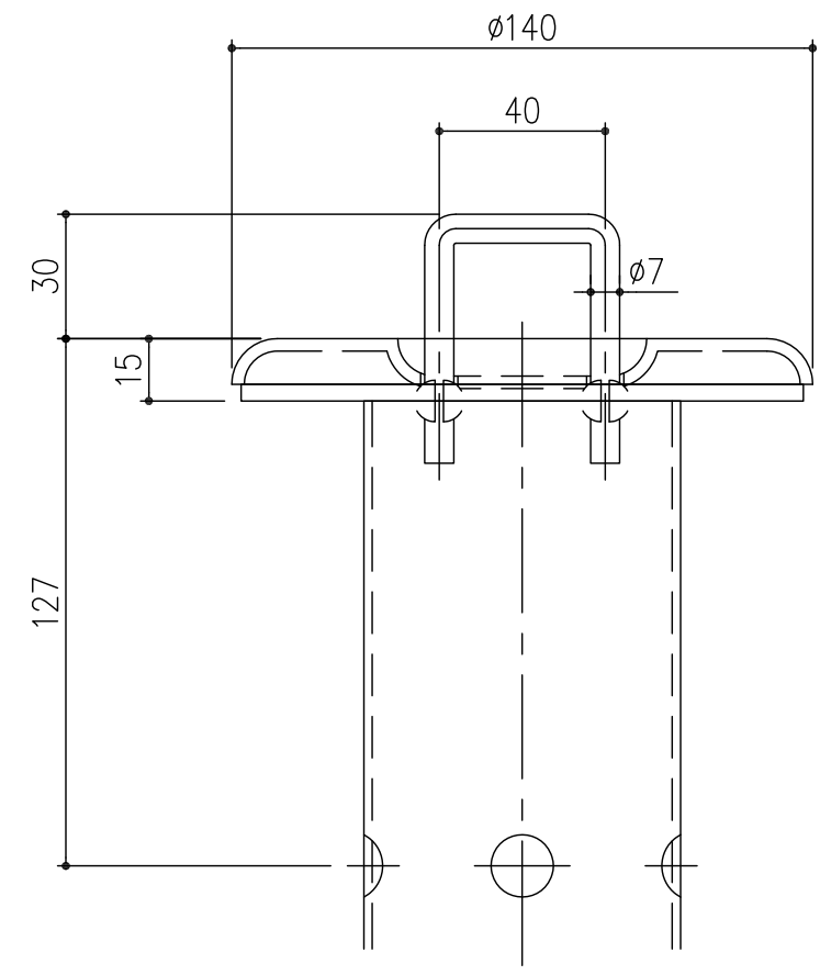
頭部詳細図 S=1/2
