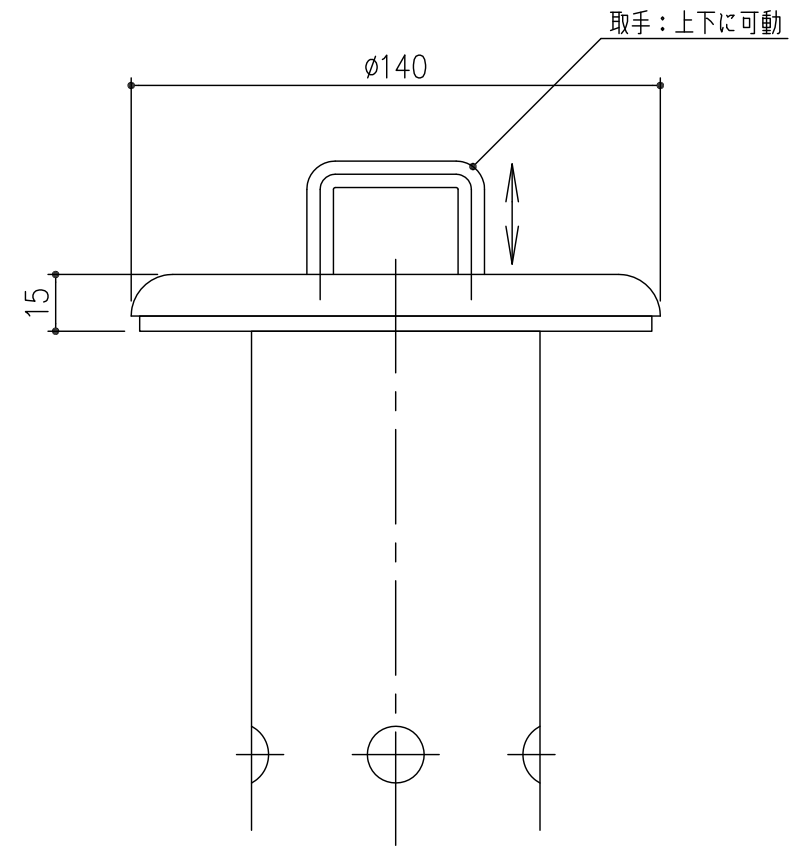
頭部詳細図 S=1/2
