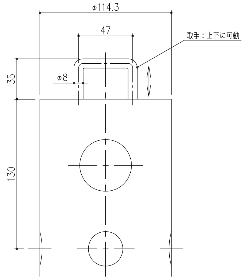
頭部詳細図 S=1/2
