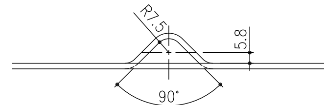
中間取付部詳細 S=1/2
