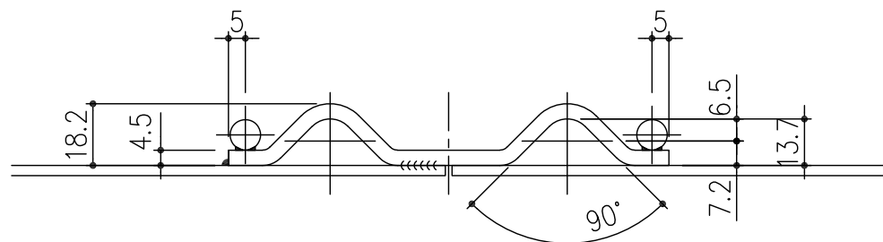
両端取付金具部詳細 S=1/2
