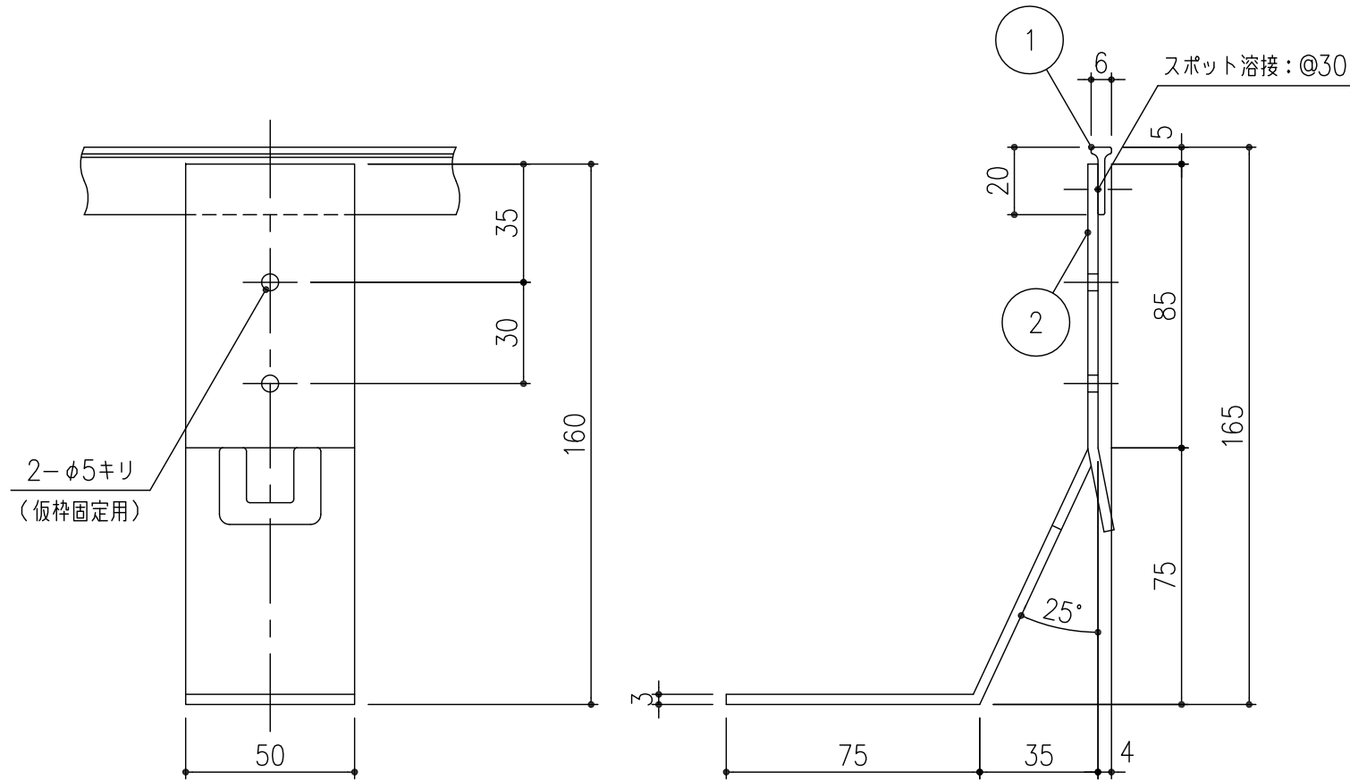
アンカー詳細 S=1/2
