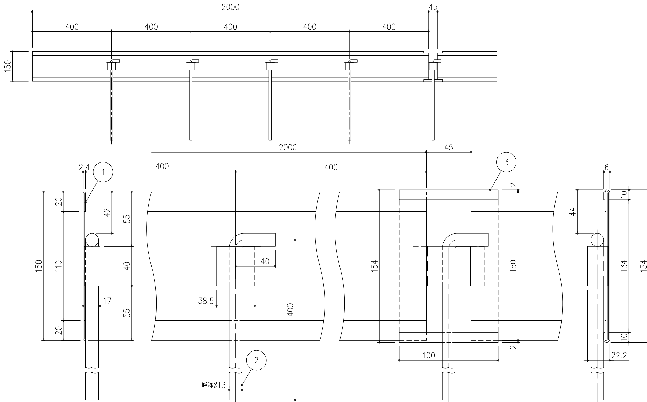
連結金具取付部詳細図 S=1/2
