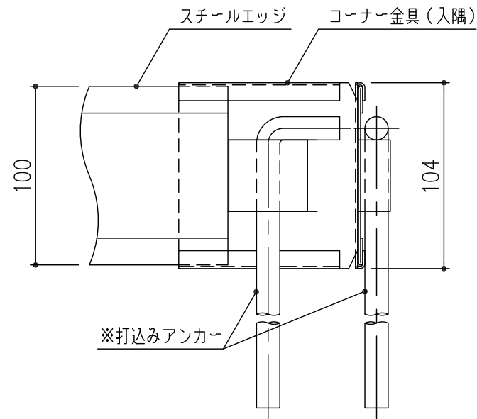
コーナー金具（入隅）
