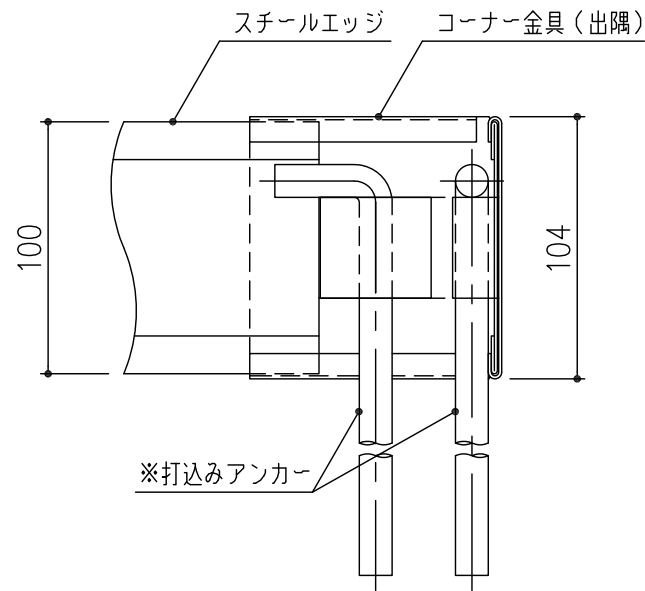
コーナー金具（出隅）
